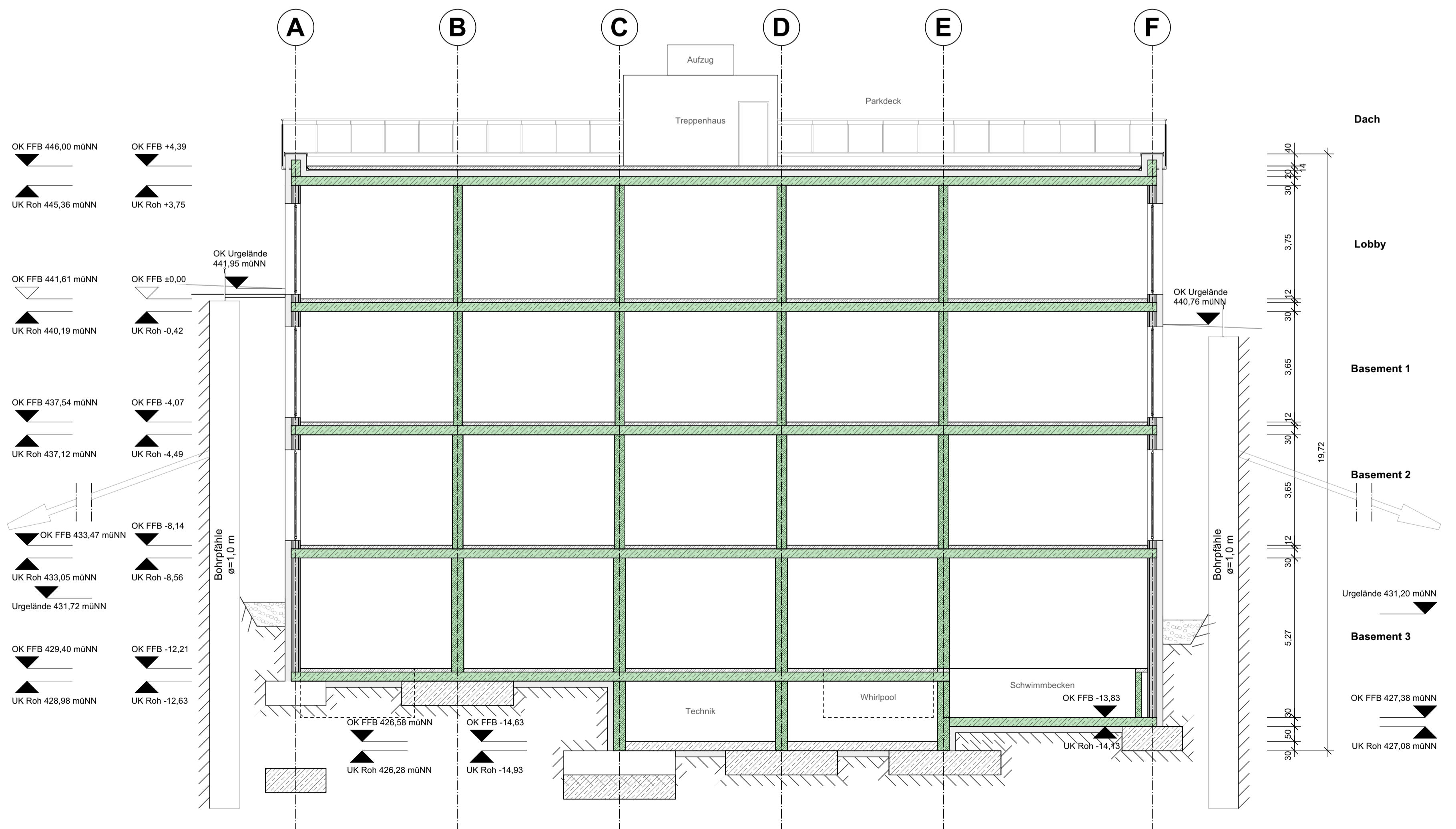
Schnitt A-A
