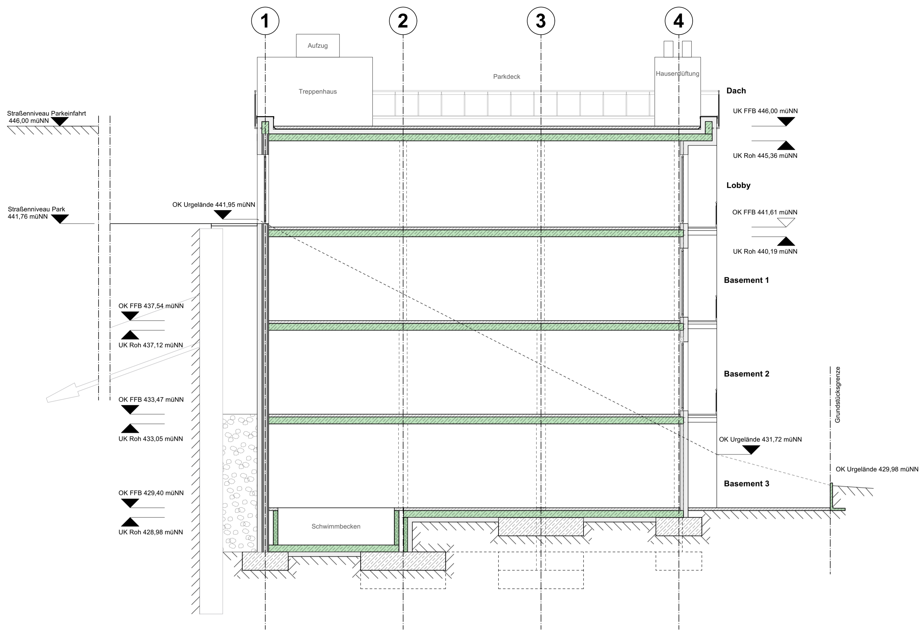
Schnitt B-B
